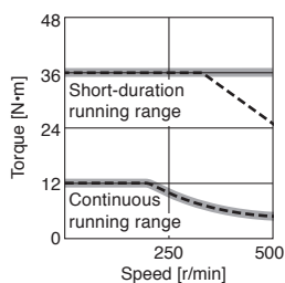
TM-RFM048G20 (Note 1, 3)
