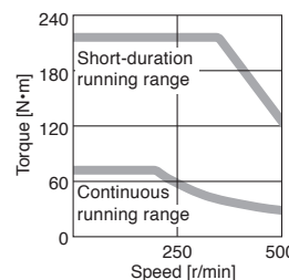
TM-RFM240J10 (Note 1, 3)
