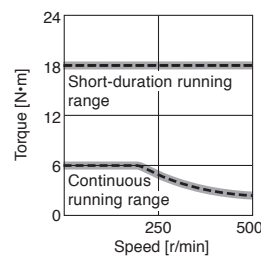
TM-RFM018E20 (Note 1, 2, 3)
