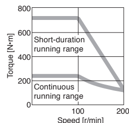
TM-RFM240J10 (Note 1, 3)
